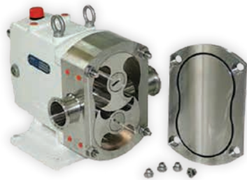
Lobe Pompa / Lobe Pump Лопастной насос / مضخة اللوب
